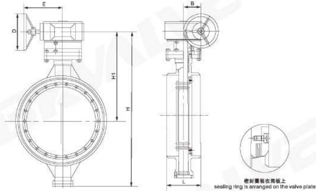
主要连接尺寸 Main connection dimensions
