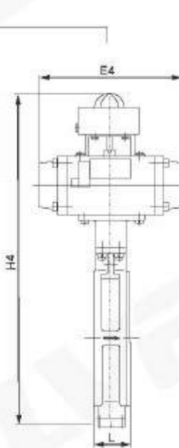
图Figure-5 气动GD675型 Pneumatic GD675
