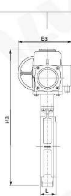
图Figure-4 电动GD975型 Electric GD975
